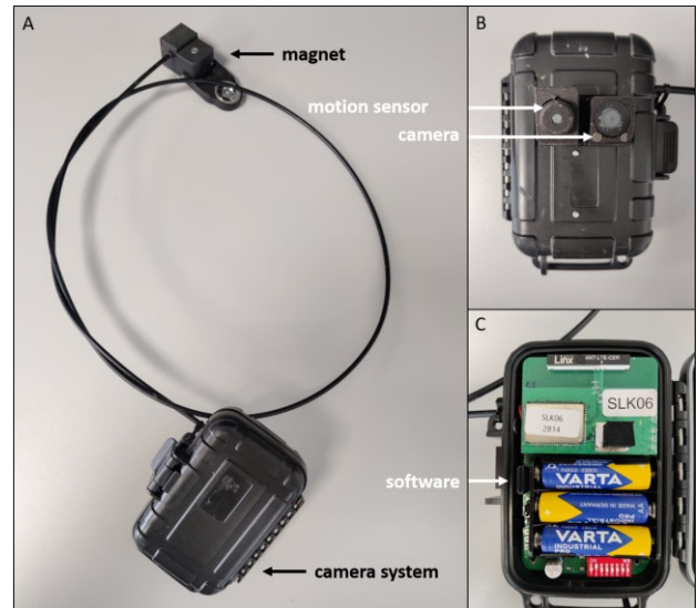
Figuur 16: Componenten van het beeldherkenningsysteem. (A) De camera is verbonden met de elektromagneet, die kan worden aangesloten op de deur van de kooi. (B) Vooraanzicht van de camera. (C) Camerasysteem en minicomputer van binnenuit.
