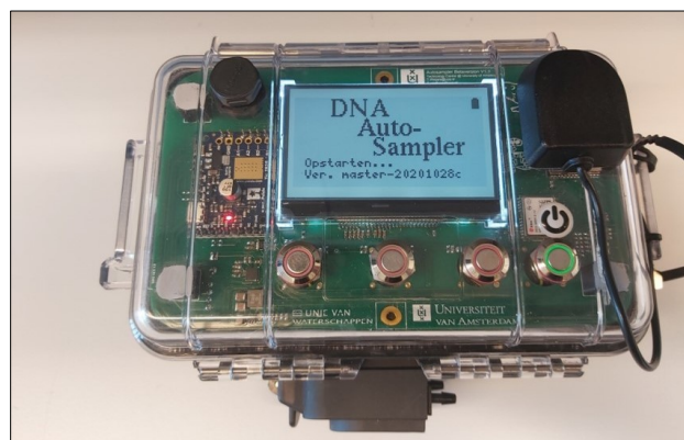
Figuur 9: eDNA autosampler voor geautomatiseerde watermonsternamen.
